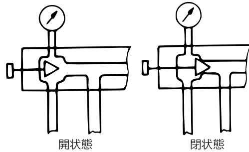
ゲージマニホールドの開閉状態
