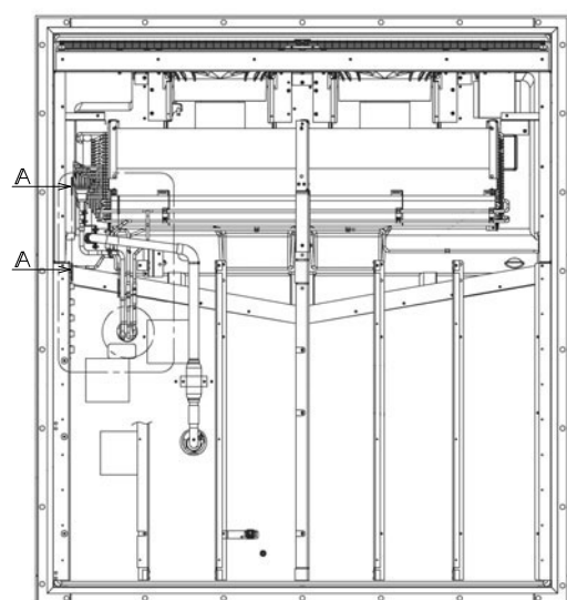
A-A断面(Section of A-A)
