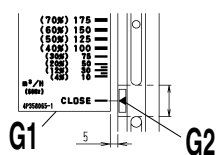
BB部詳細
